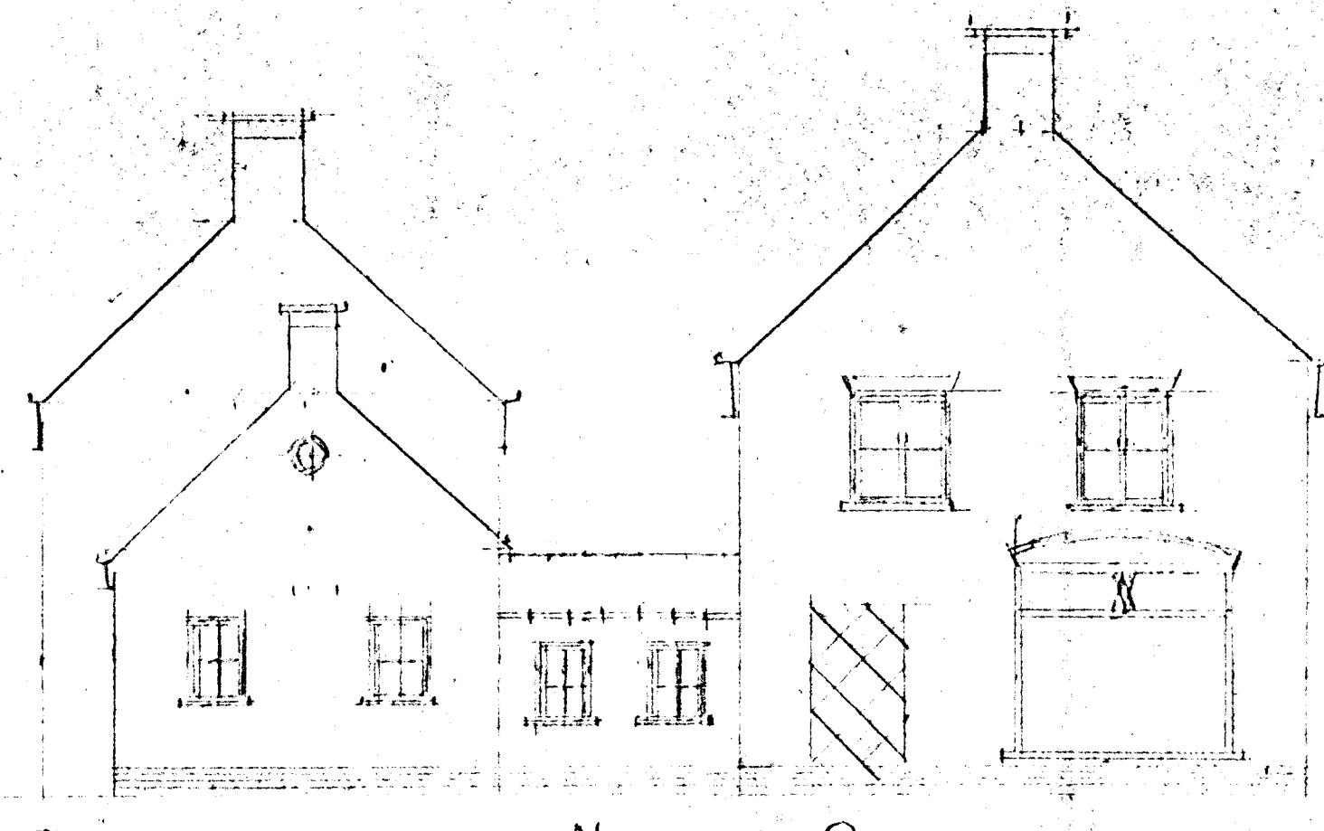
BESTAANDE, TEVENS NIEUWE OOSTGEVEL
