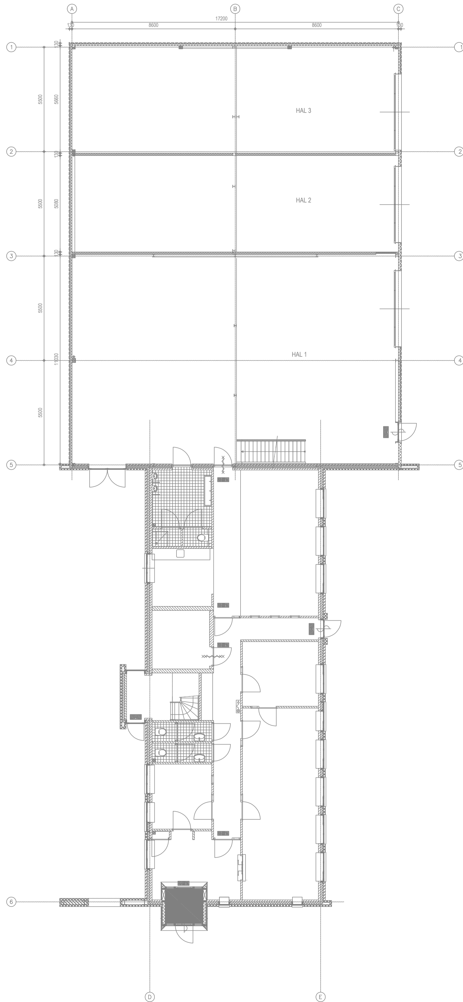
PLATTEGROND BEGANE GROND
