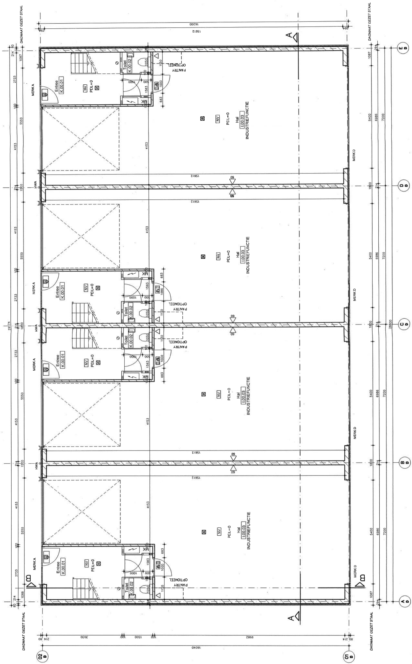
PLATTEGROND BEGANE GROND (bouwdeel D/E) PEIL=0
