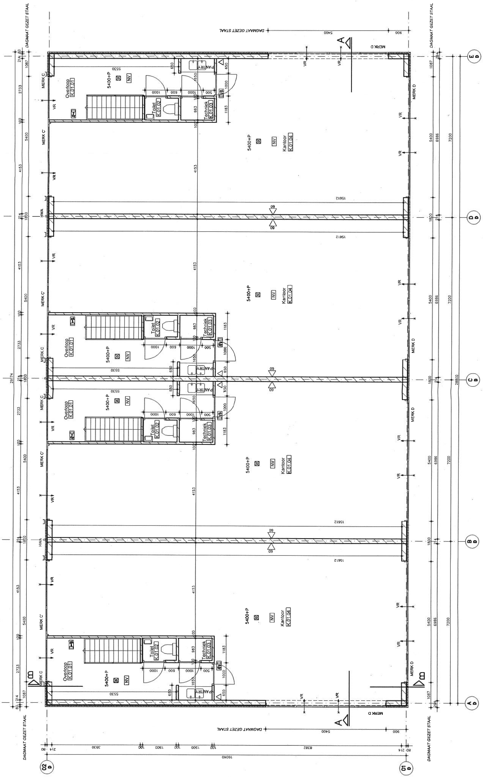
PLATTEGROND VERDIEPING (bouwdeel D/E) PEIL=5400+
