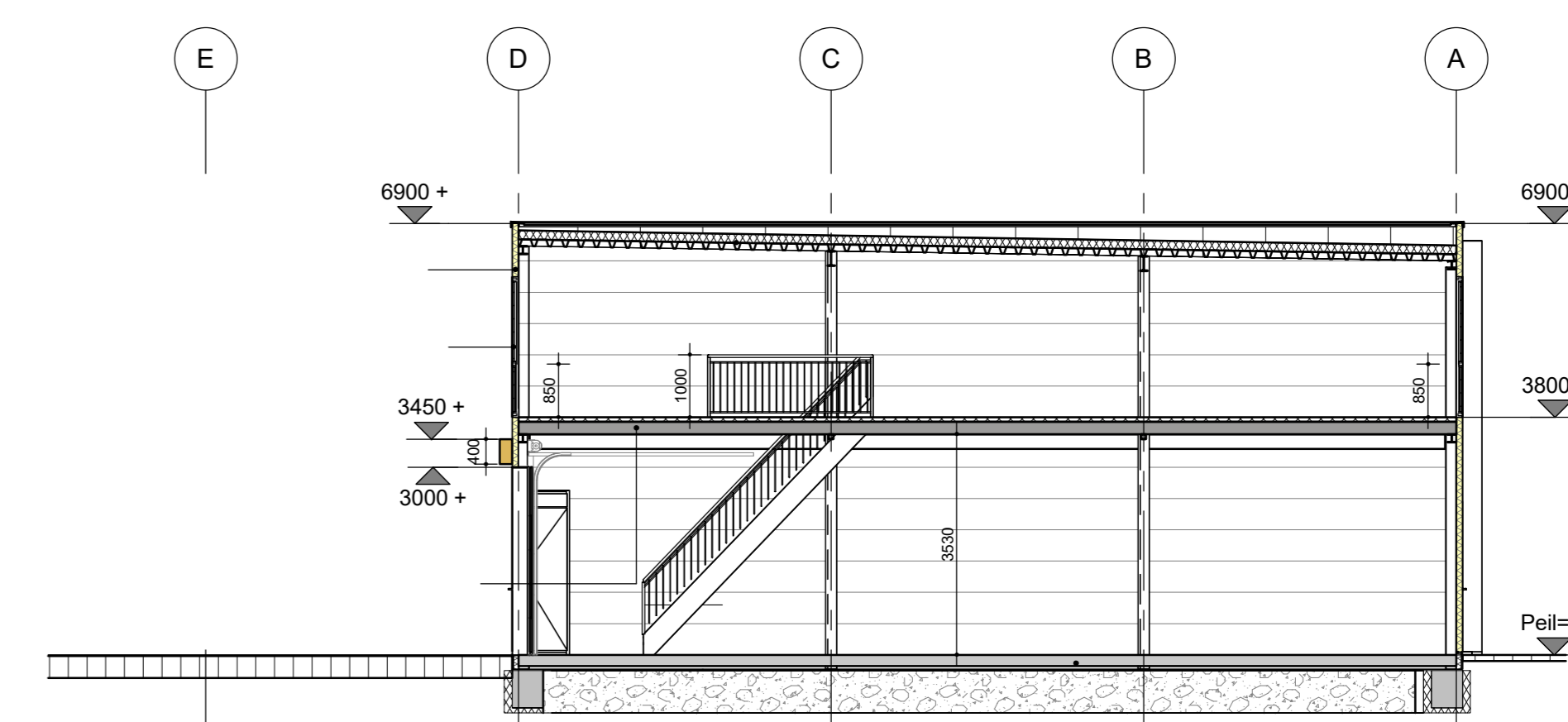
Doorsnede B-B
