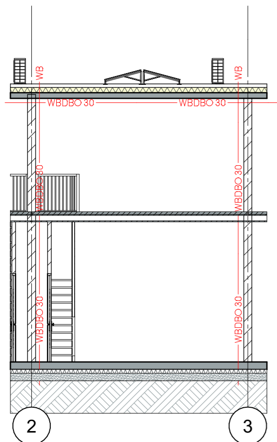
Doorsnede C
