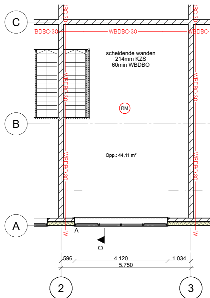
1e verdieping
