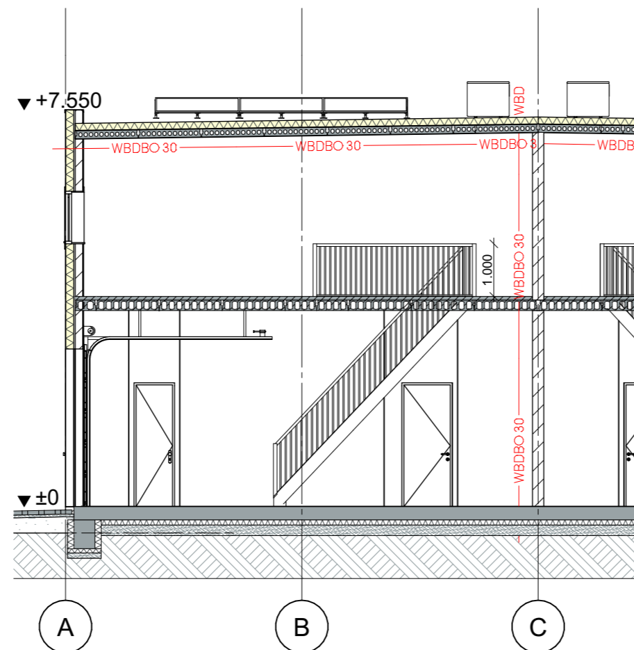
Doorsnede D
