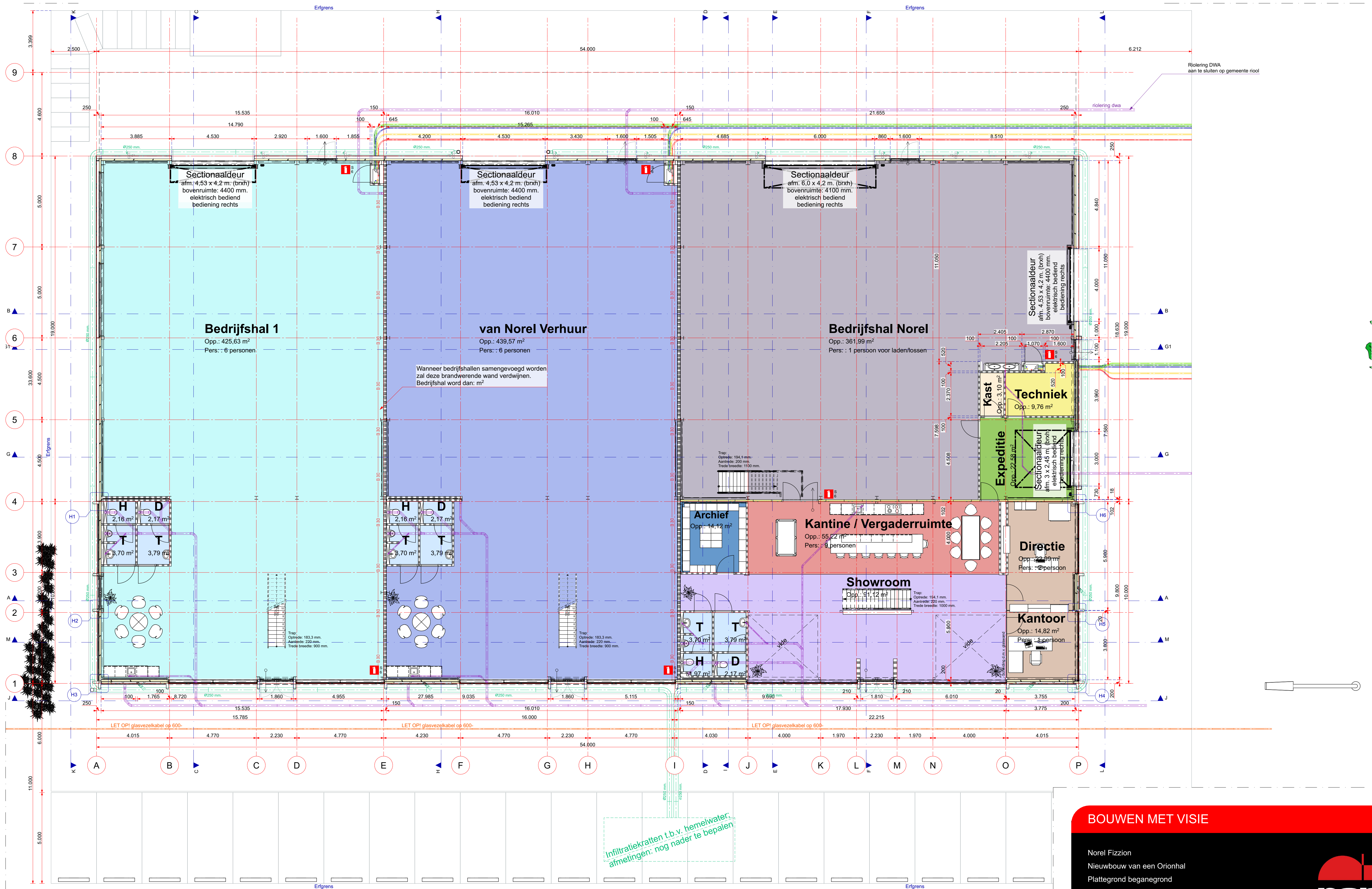
Plattegrond beganegrond
